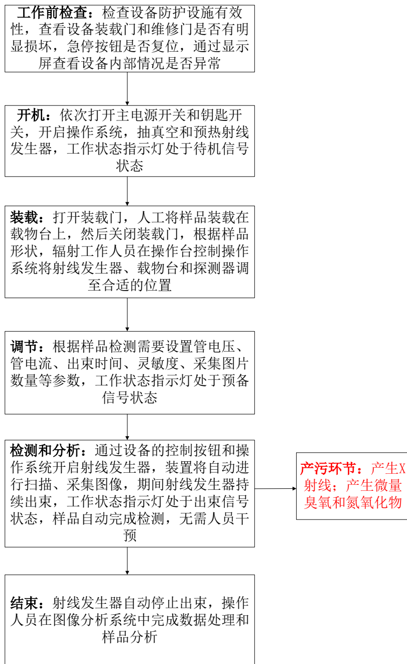
图 2-8 操作流程和产污环节图
