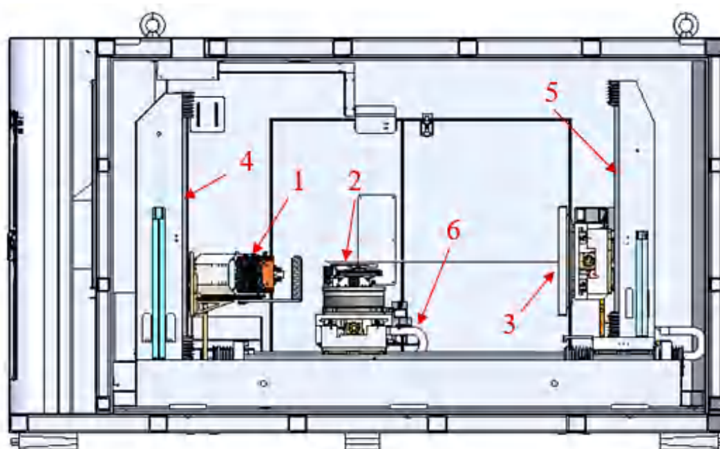
图 2-6 工业 CT 内部结构图
