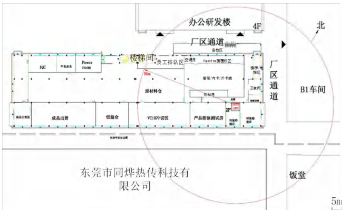
图 2-3 B2 车间一层平面布置图
