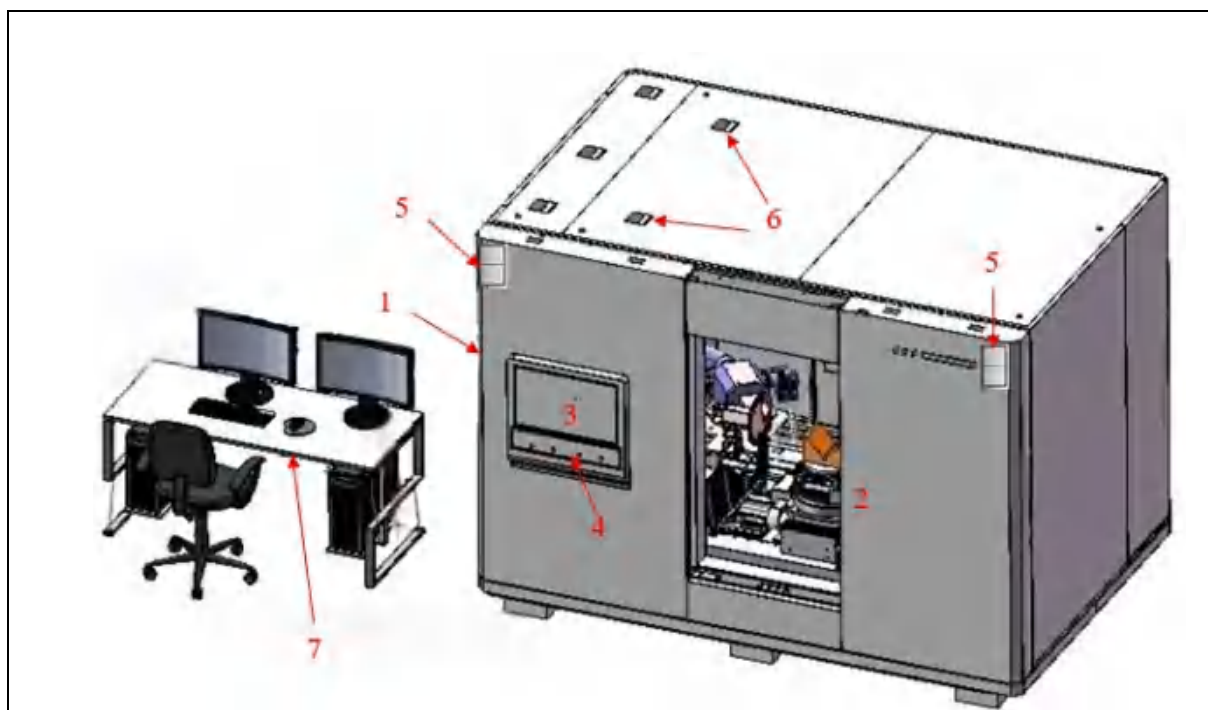
图 2-5 工业 CT 外观结构图
