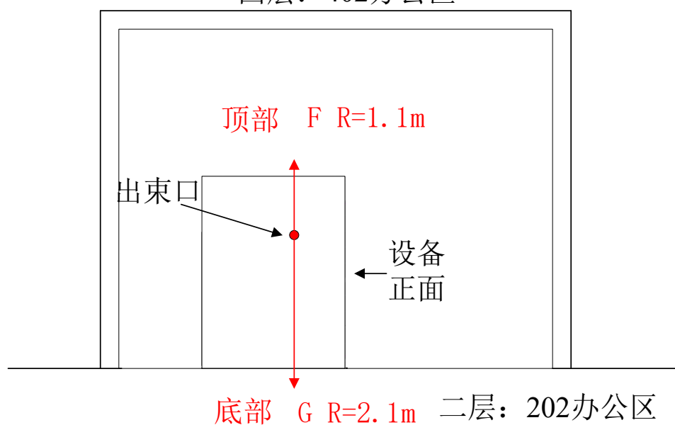
图 11-3 关注点分布示意图（立面）
