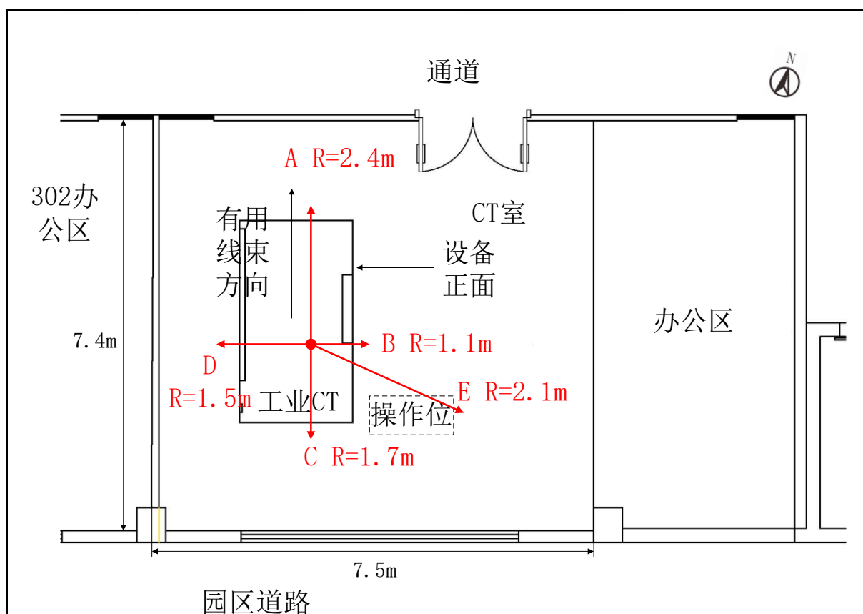
图 11-2 关注点分布示意图（平面）
