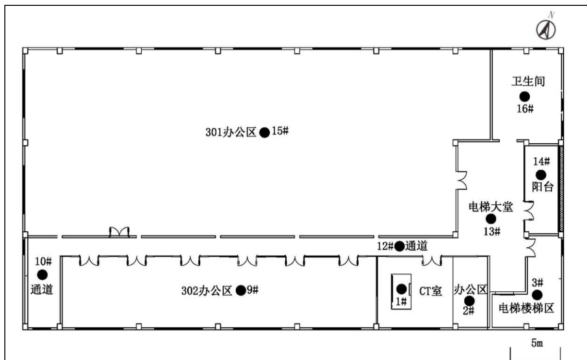
图 8-3 3 层检测布点图
