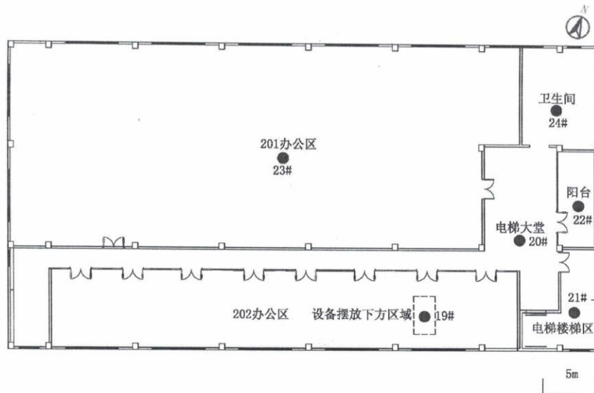
2 层检测布点图
