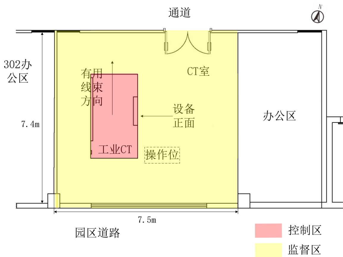
图 10-8 辐射工作场所布局和分区示意图
