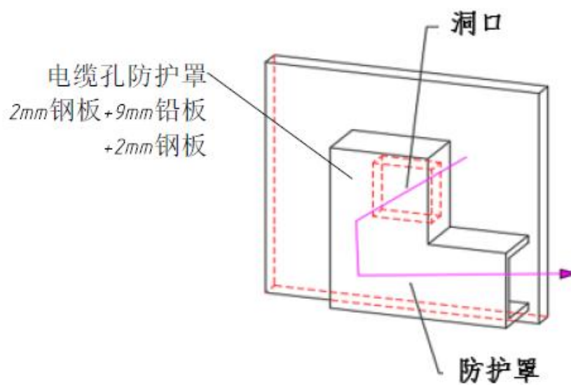
图 10-4 电缆孔穿屏蔽体示意图
