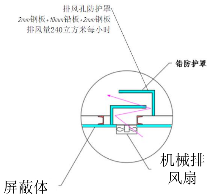
图 10-5 排风口屏蔽示意图
