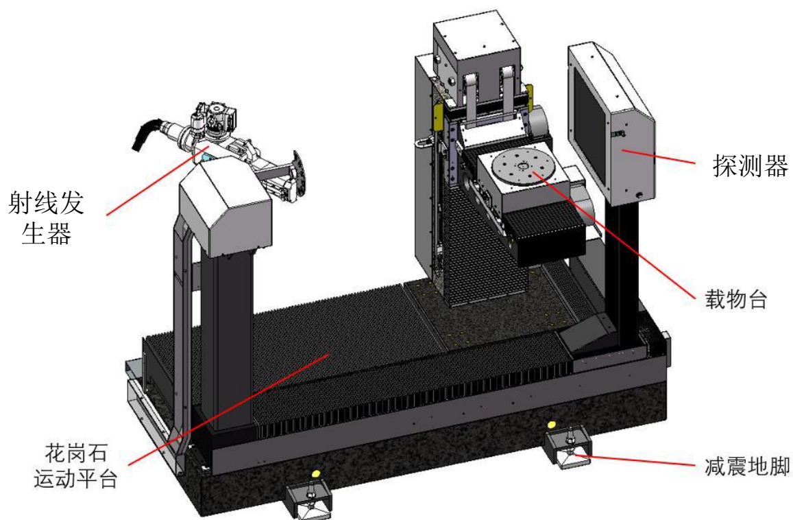
图 9-2 工业 CT 内部结构图
