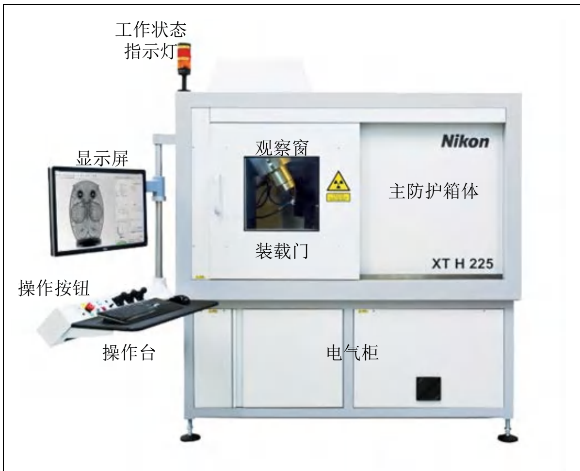
图 2-4 工业 CT 外观结构图
