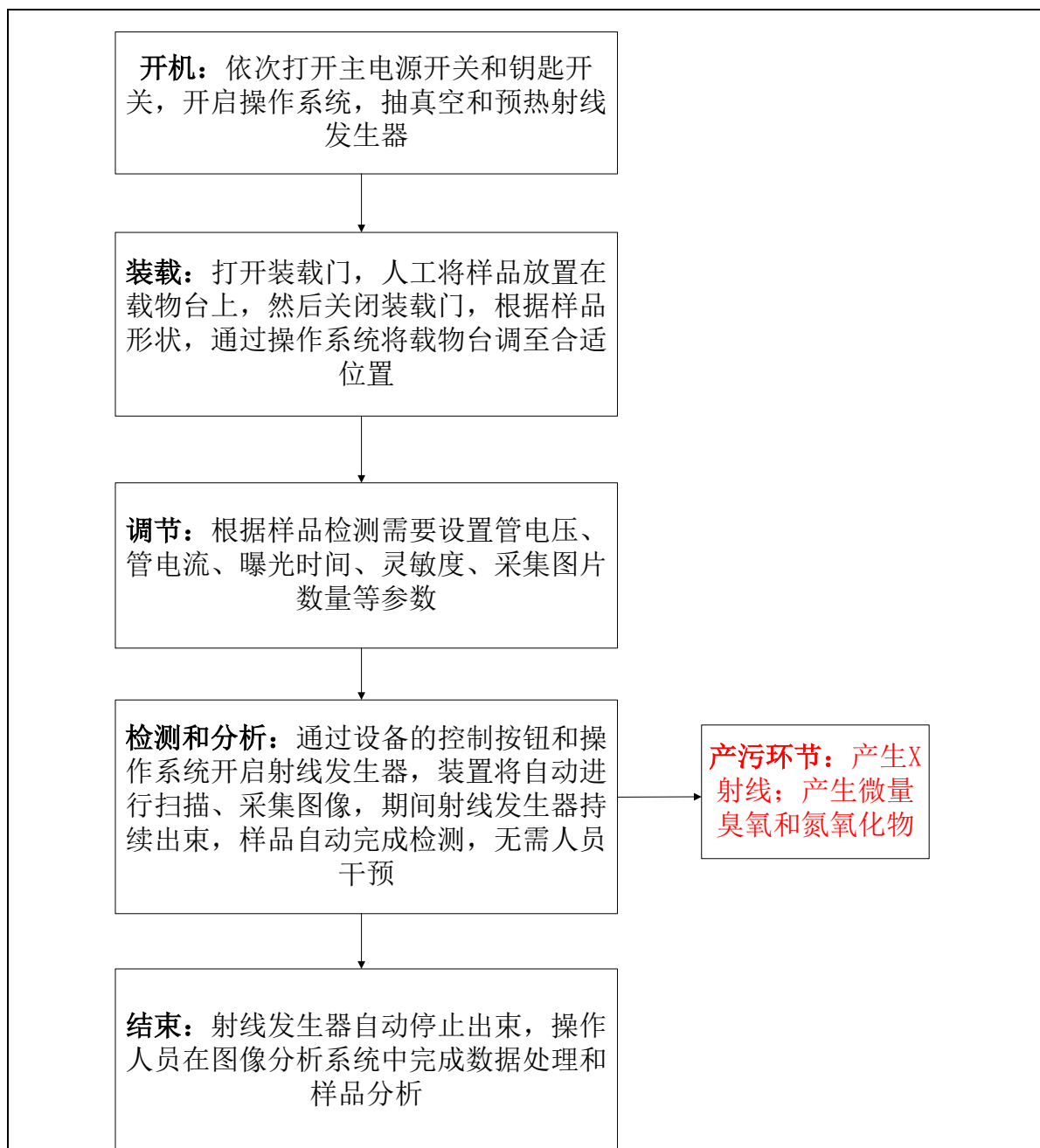
图 2-7 操作流程和产污环节图
