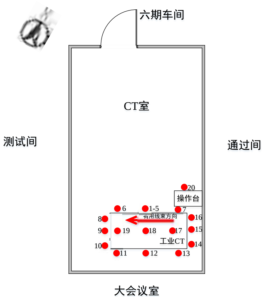
图 6-1 监测布点图
