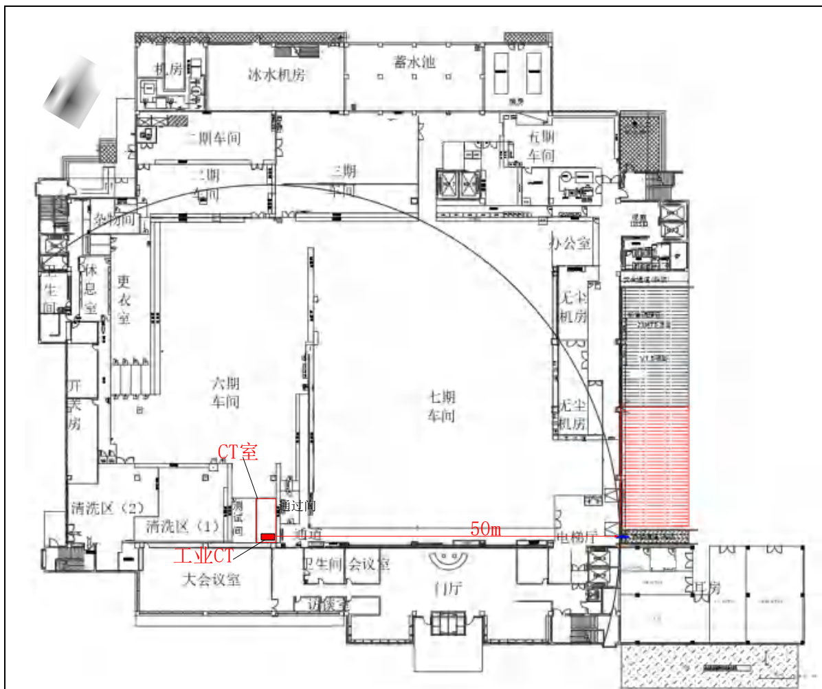
图 2-3 一期厂房一层平面布置图
