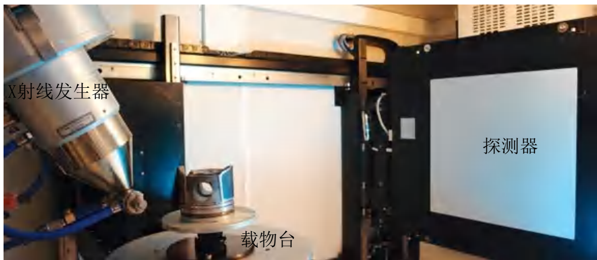
图 2-5 工业 CT 内部结构图
