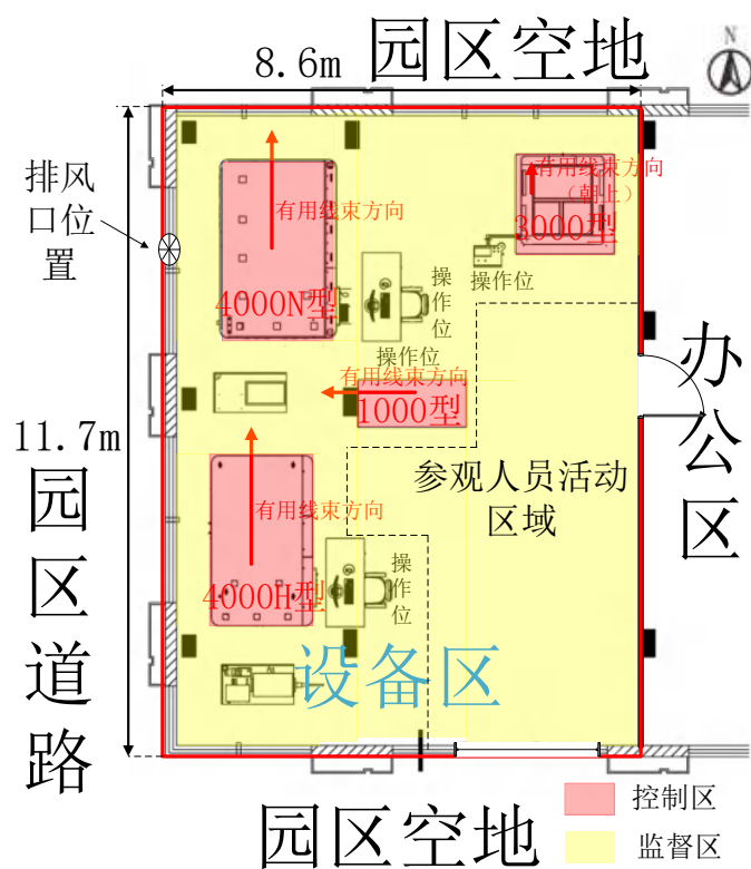
环评辐射工作场所布局和分区示意图
