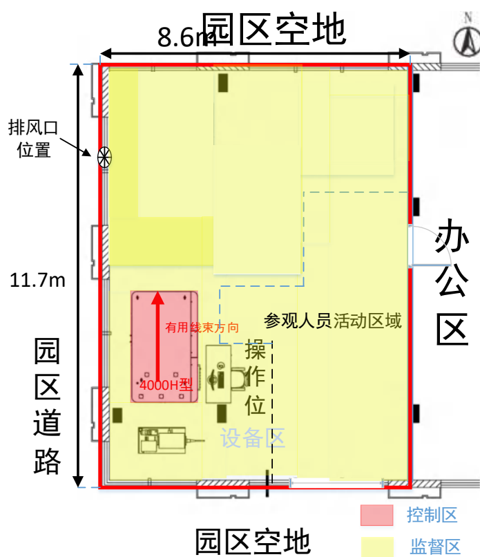
实际辐射工作场所布局和分区示意图
