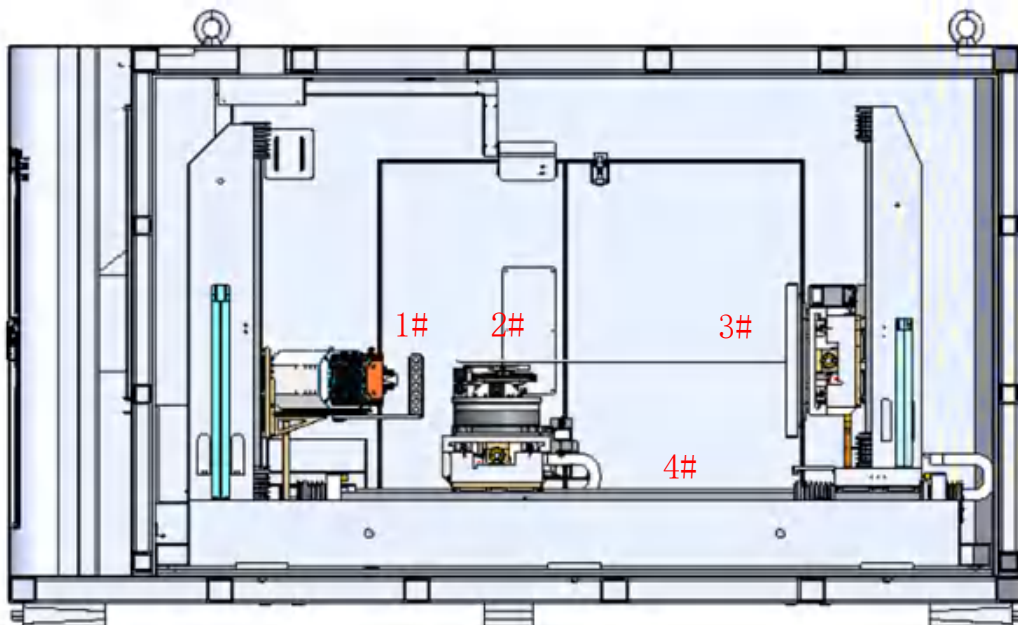
图 2-6 设备内部结构图
