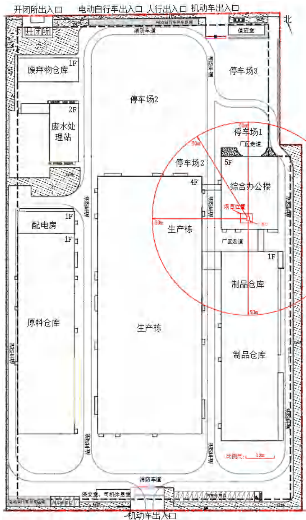
图 2-2 东丽佛山公司平面布置图
