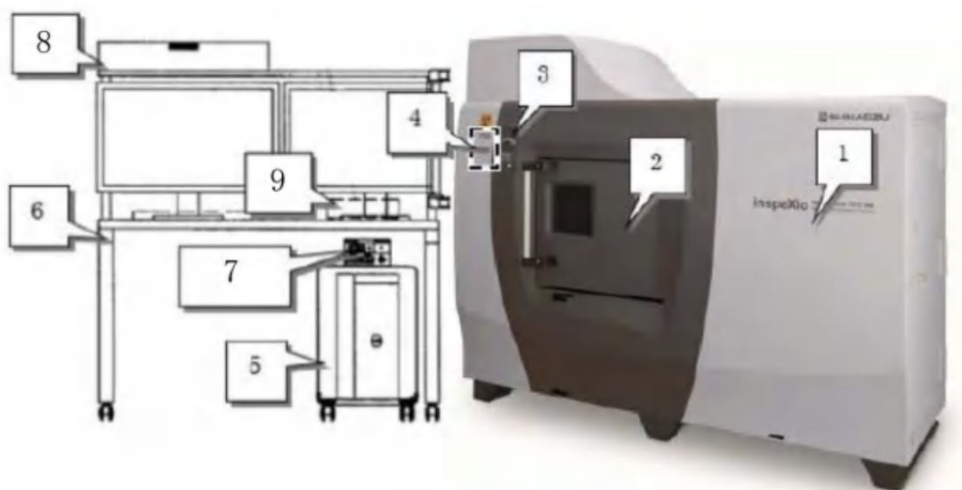
图 2-5 工业 CT 外观结构图
