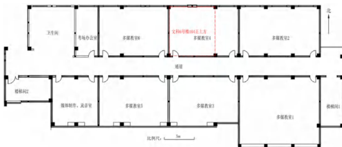
图 2-5 三峡大学文科 6 号楼二层平面布置图
