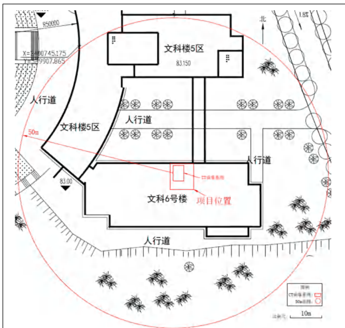
图 2-3 三峡大学文科 6 号楼四周平面布置图及项目周边 50m 关系图
