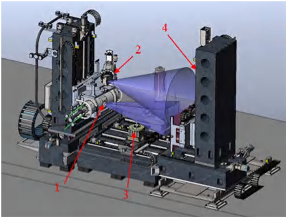
图 2-7 CT 成像系统内部结构图
