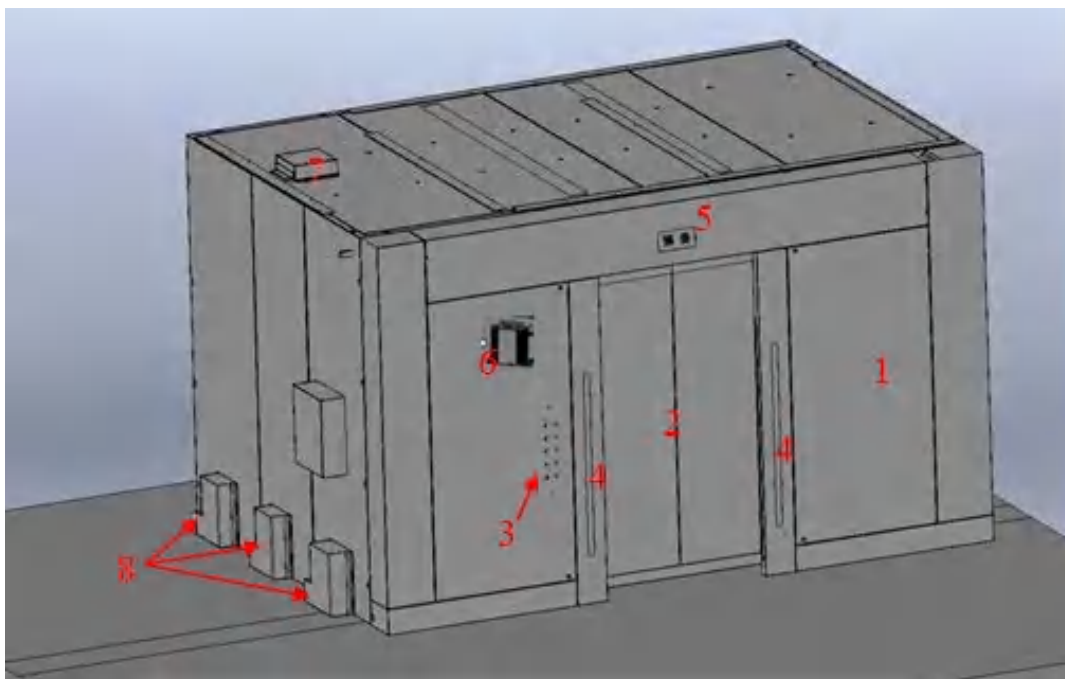
图 2-6 CT 成像系统外观结构图
