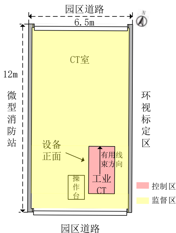
图 3-1 工作场所布局和分区示意图
