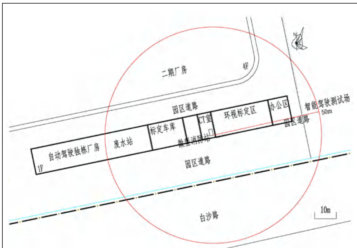
图 2-3 自动驾驶独栋厂房平面布置图和项目周边 50m 关系图
