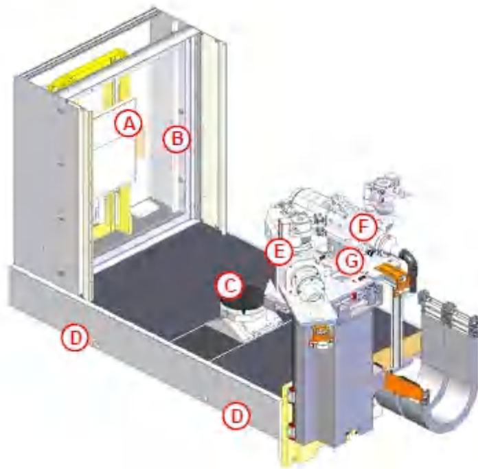
图 2-6 设备内部构造示意图
