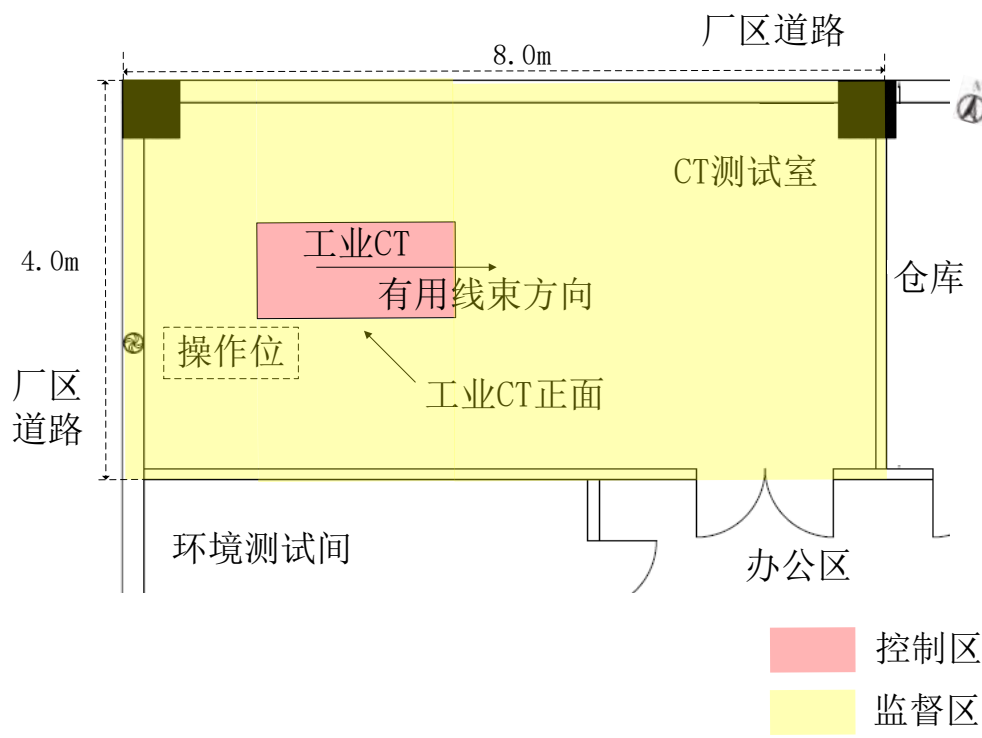
图 3-1 工作场所布局和分区示意图
