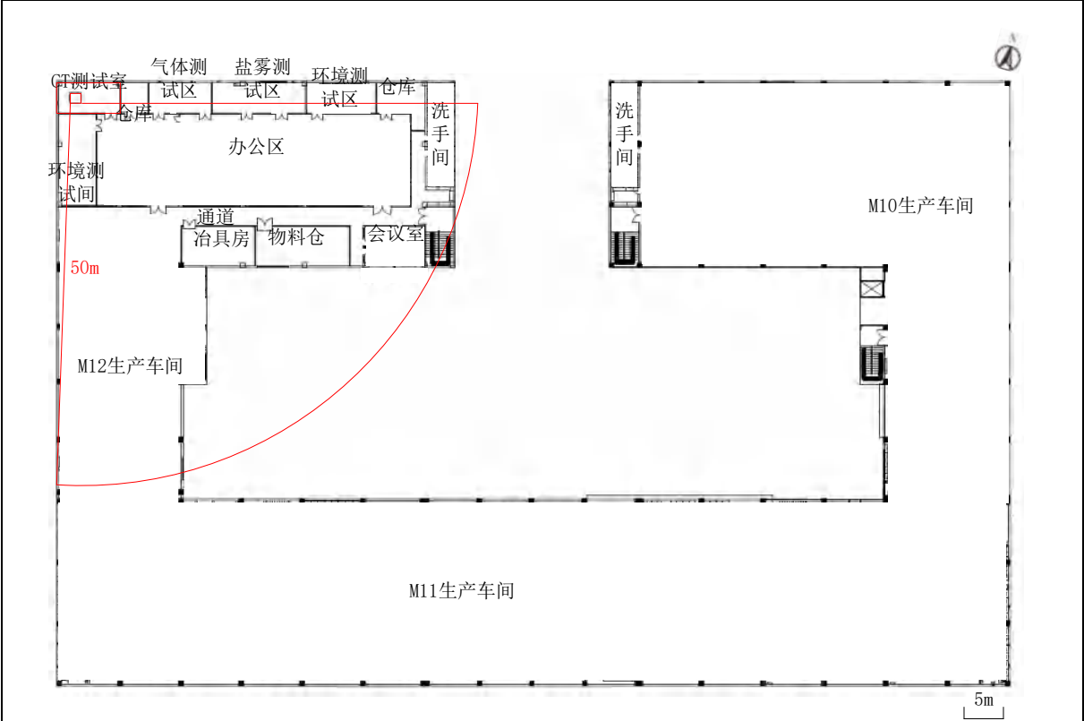
图 2-39 栋 2 层平面布置图
