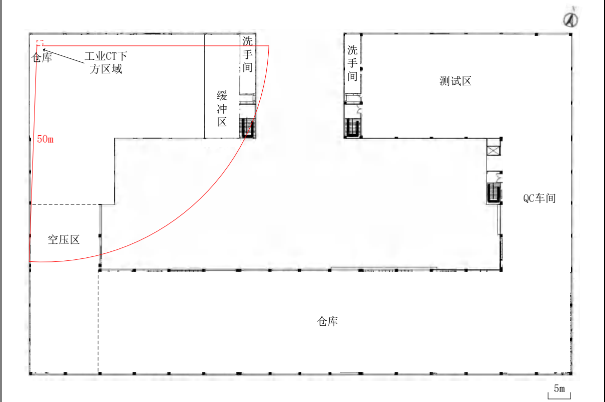
图 2-49 栋 1 层平面布置图
