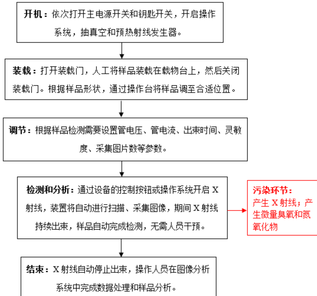
图 2-8 工艺流程和产污环节图
