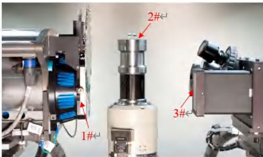
图 2-6 工业 CT 内部结构图
