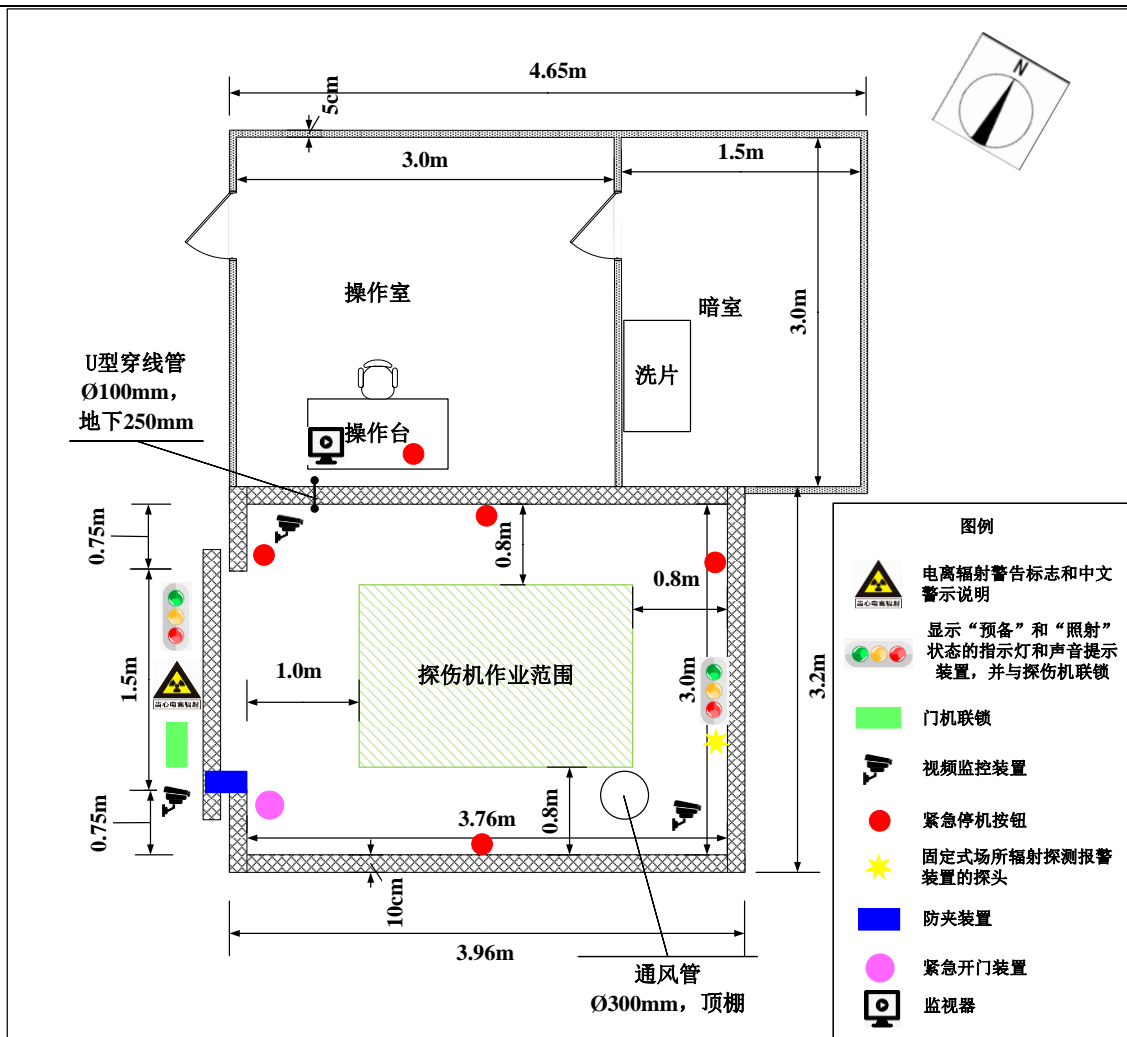
图 10-4 本项目探伤室辐射安全和防护设施布置图
