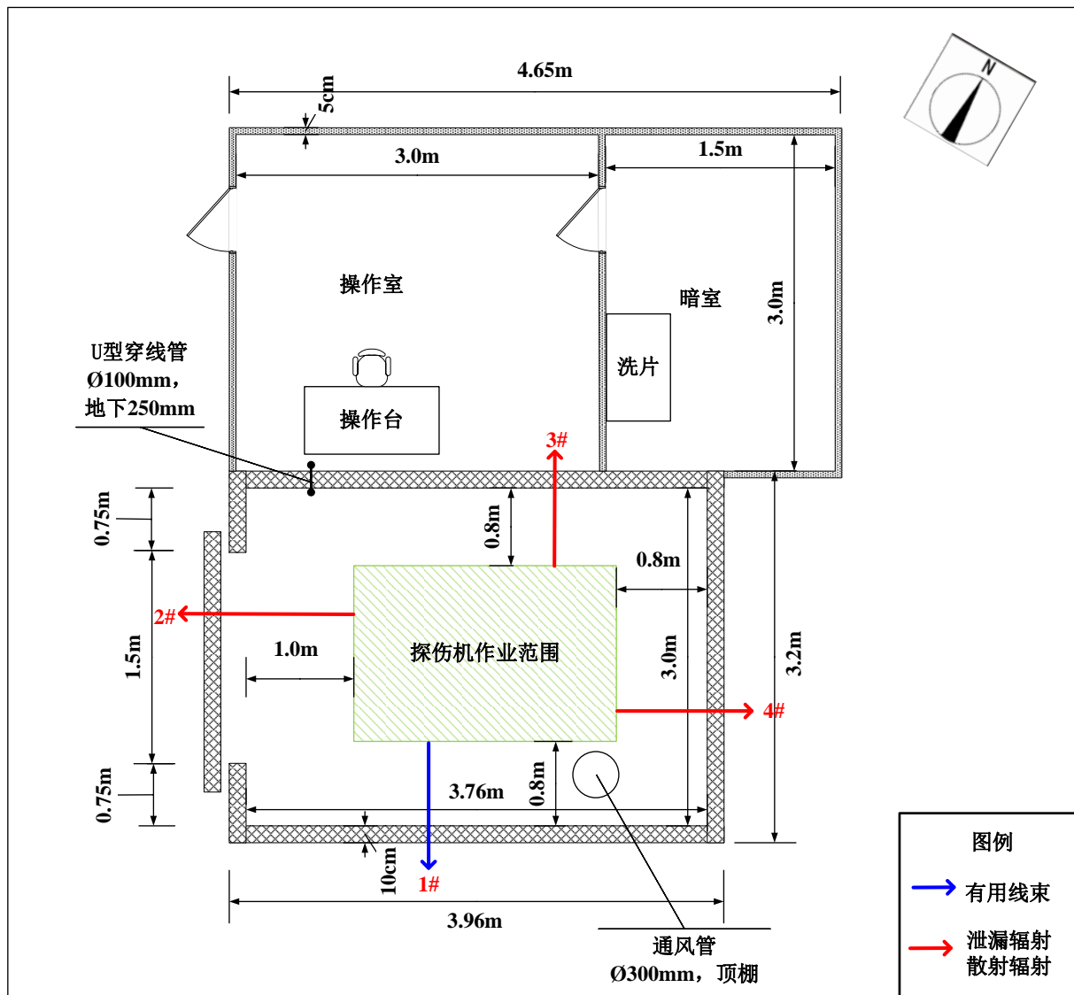
图 11-1 探伤室平面布局及周围环境预测点位示意图
