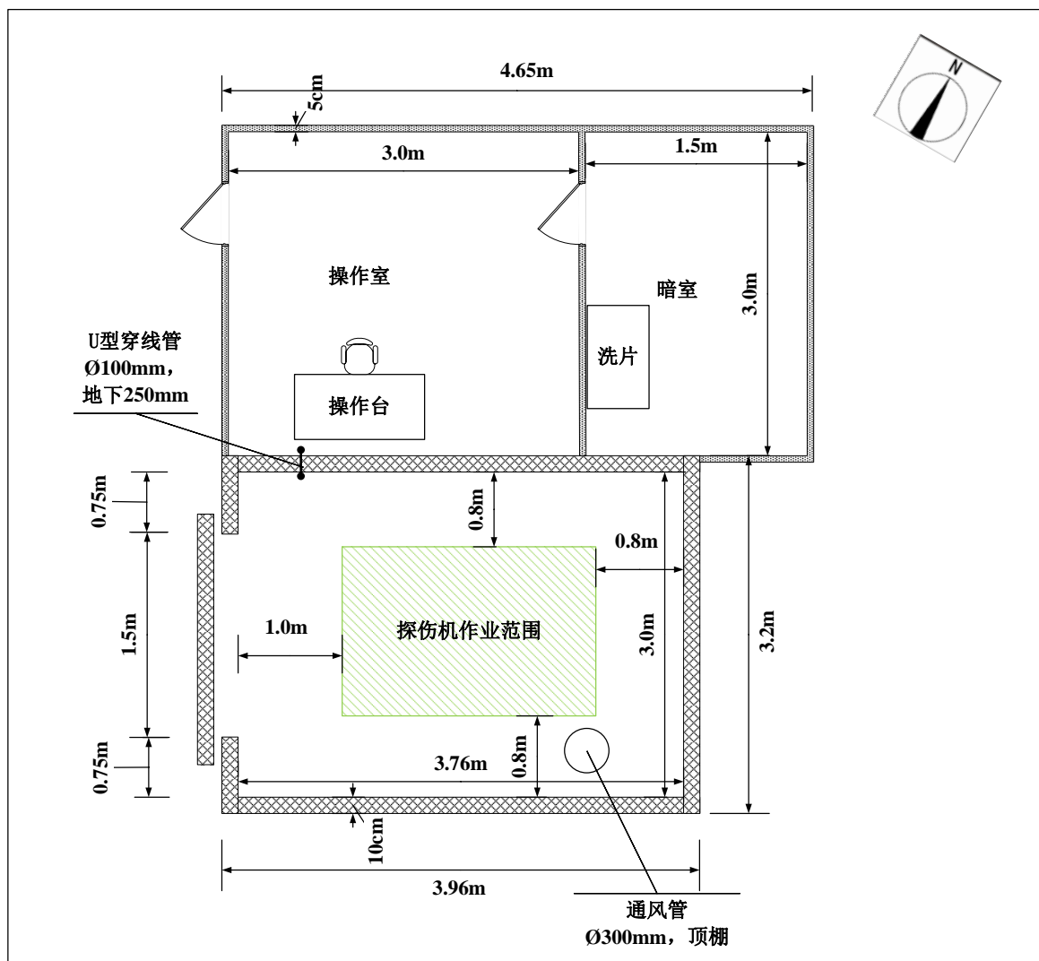
图 10-2 本项目探伤室平面设计示意图
