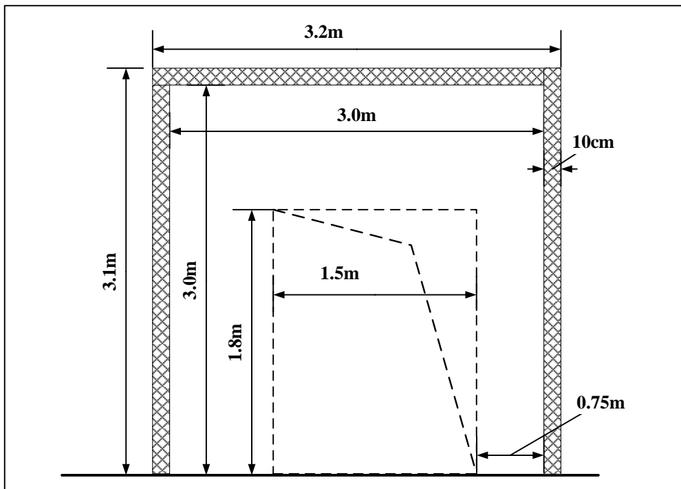
图 10-2 本项目探伤室剖面图
