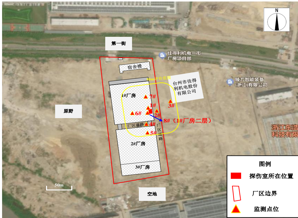
图 8-1 本项目探伤室监测点位分布图
