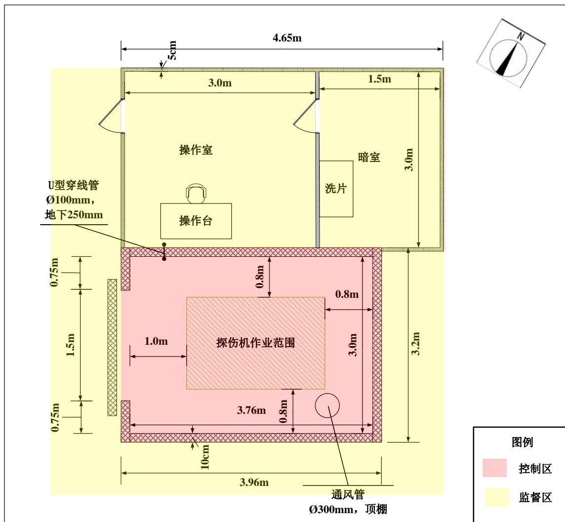
图 10-1 本项目探伤工作场所分区管理示意图
