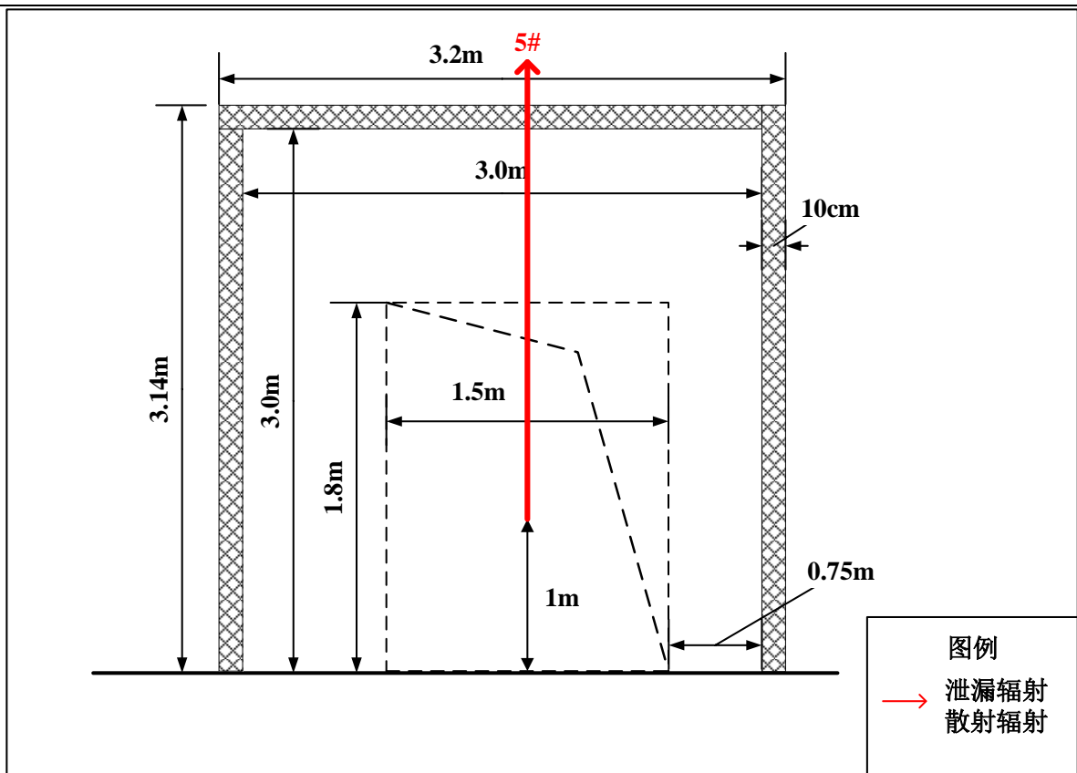
图 11-2 探伤室剖面布局及周围环境预测点位示意图
