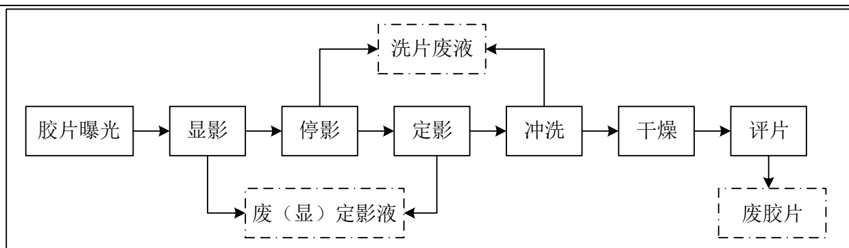
图 9-5 洗片室洗片工艺流程及产污环节示意图
