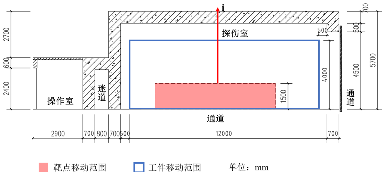
图 11-2 本项目探伤室剖面布局与预测点位图
