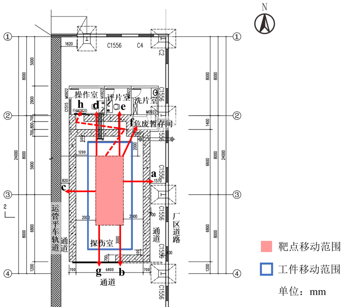
图 11-1 本项目探伤室平面布局与预测点位图
