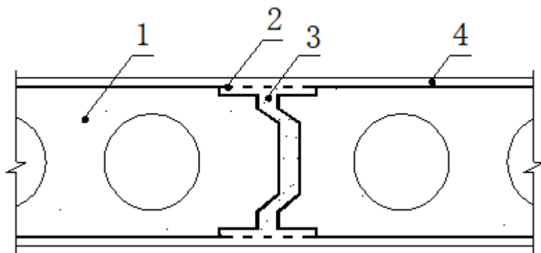
图5.2.1 GRC板连接示意图
