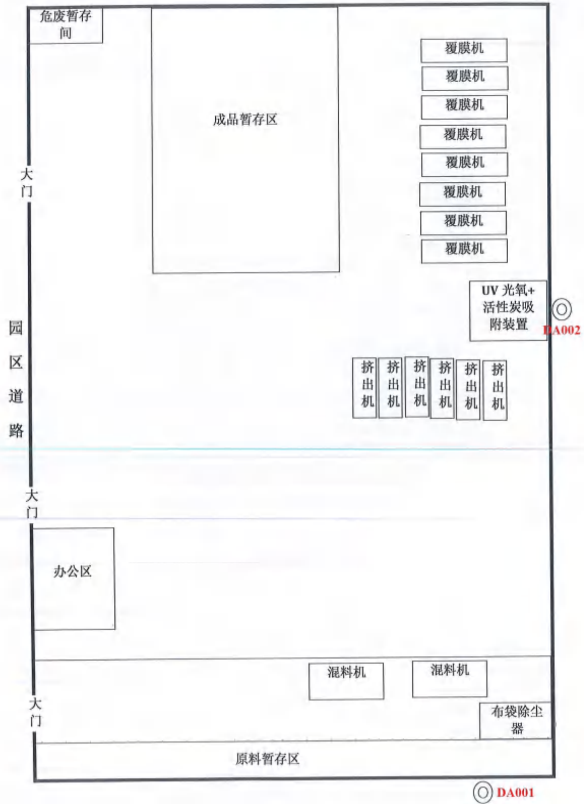
附图 3 项目车间平面布置图
