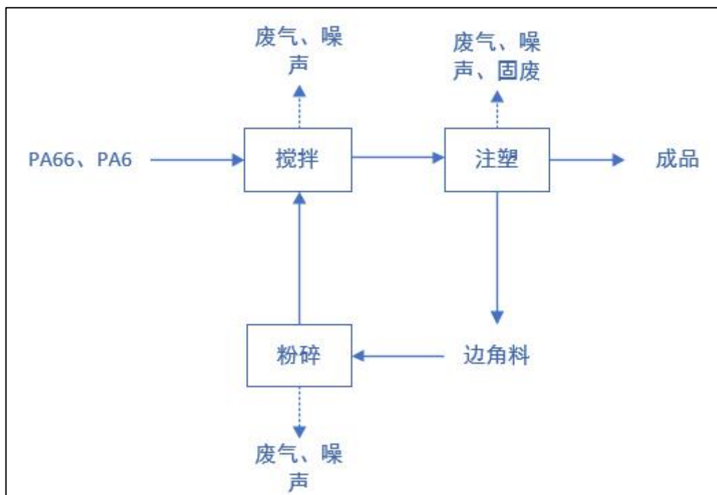
图 2-4 主要工艺流程及产污环节图
